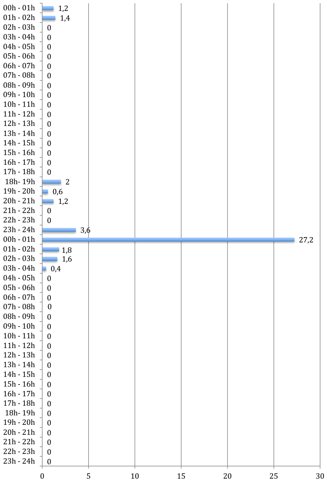
Cantidades de lluvia registradas por horas en OROPESA DEL MAR el día 01 y 02/09/21 (en l/m²)
